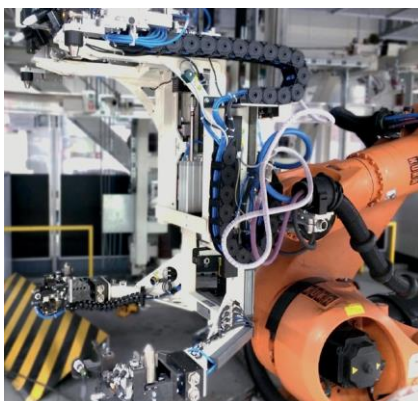
>> Greifer für Frontend fügen
