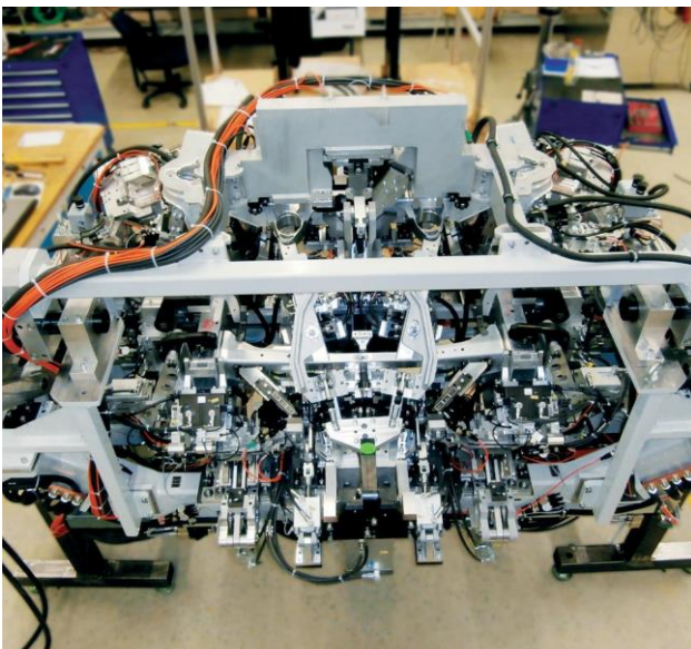
>> Roboterschweißvorrichtung
