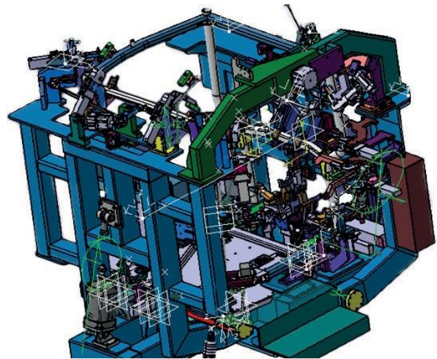
>> CAD-Modell Endschweißvorrichtung Führerhauskabine
