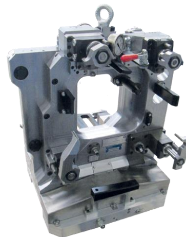
>> Spannvorrichtung: Druckgussteil
