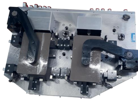
>> Spannvorrichtung Druckgussteil
