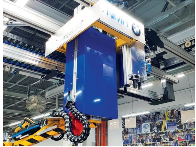
>> Handlingsgerät PKW Batterien
