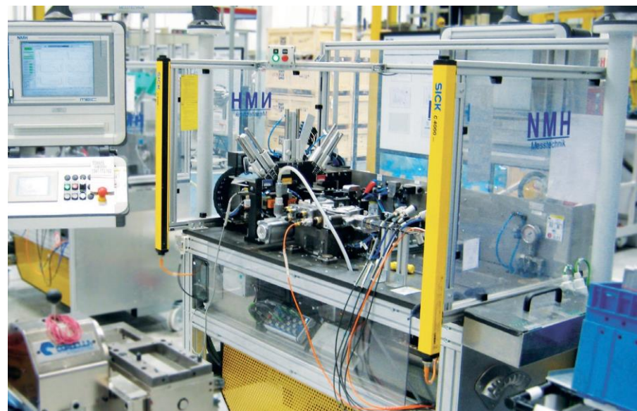
>> Messanlage zum Prüfen von Schaltauslegern im NKW Bereich
