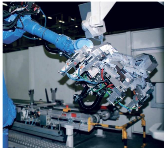
>> Robotergreifer als MIG/MAG-Schweißvorrichtung
