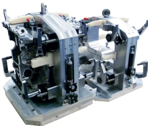
>> Spannvorrichtung: Druckgussteil
